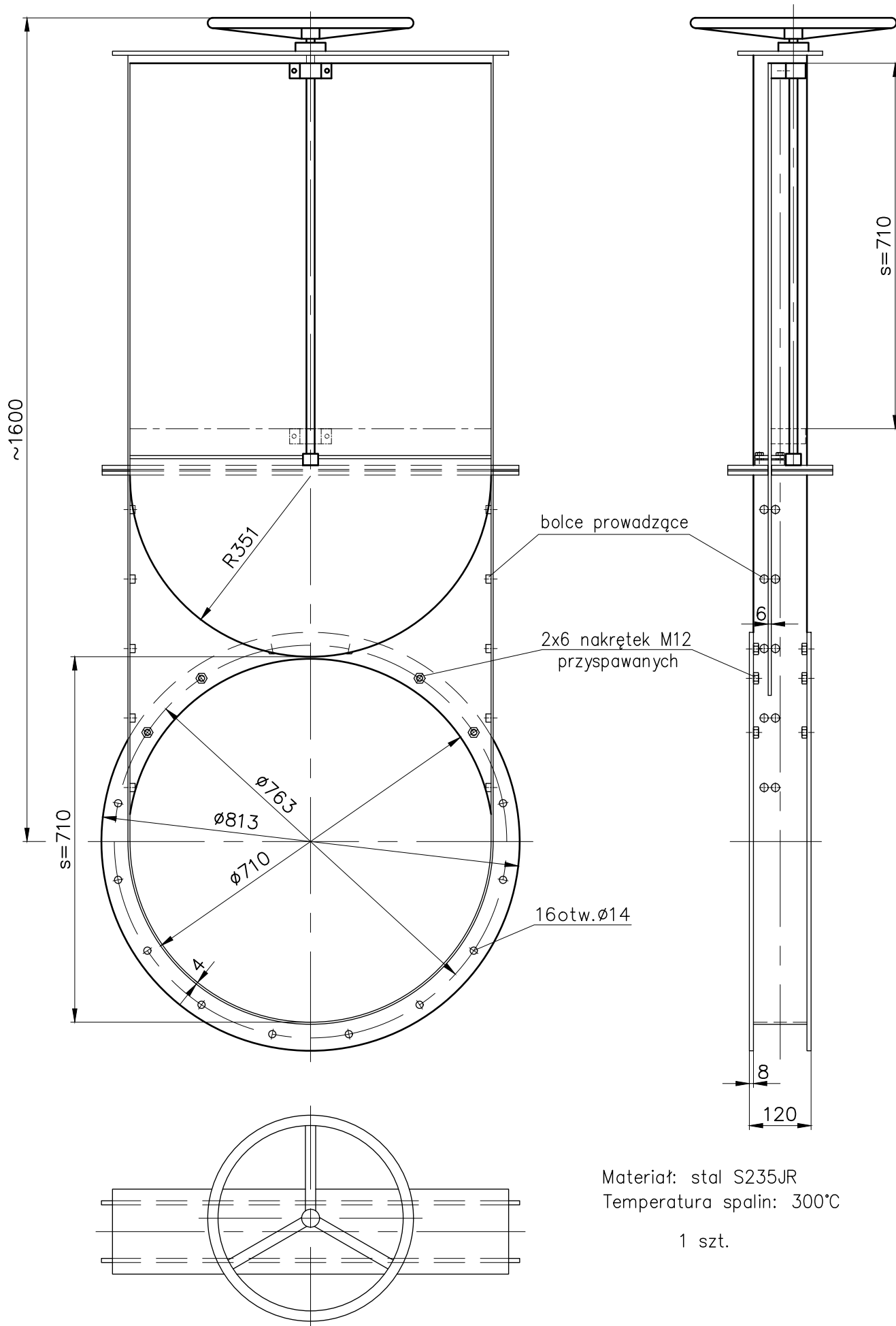
Zasuwa \phi 710 – rysunek założeniowy
